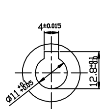
INPUT SHAFT
