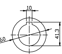
INPUT SHAFT
